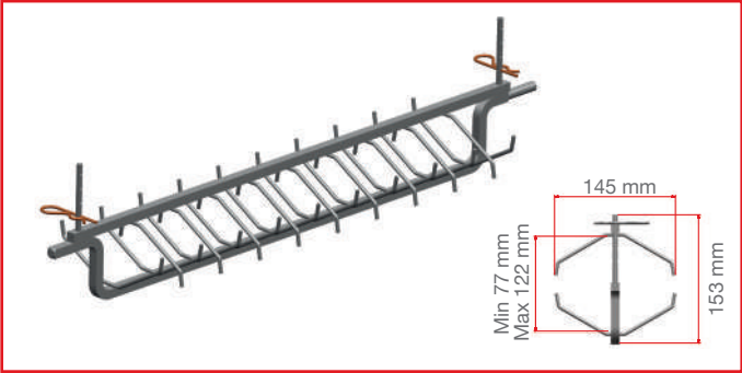
Attrezzo per arrosto
