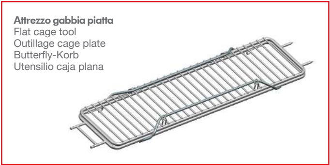
Cod. 14080146.CM Misura utile di cottura 570 mm Usable measure of cooking 570 mm Mesure utile de cuisson 570 mm Nutzbreite 570 mm Medida útil de cocción 570 mm
