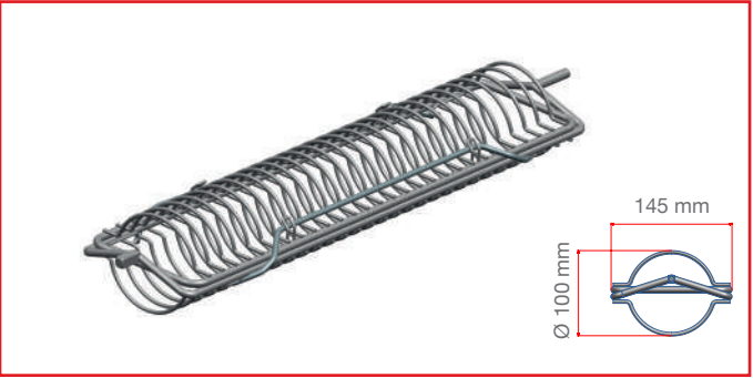
Attrezzo per arrosto Ø 100 mm
