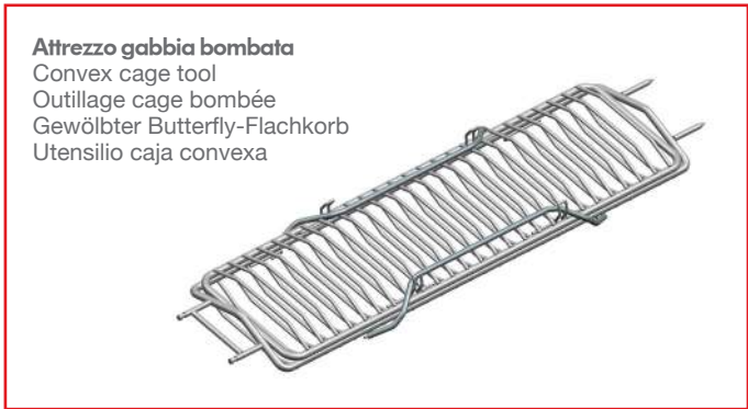
Cod. 14080508.CM Misura utile di cottura 570 mm Usable measure of cooking 570 mm Mesure utile de cuisson 570 mm Nutzbreite 570 mm Medida útil de cocción 570 mm
