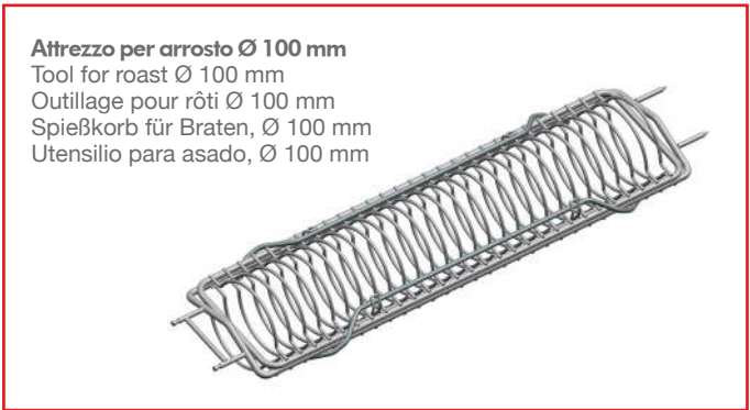
Cod. 14080507.CM Misura utile di cottura 570 mm Usable measure of cooking 570 mm Mesure utile de cuisson 570 mm Nutzbreite 570 mm Medida útil de cocción 570 mm
