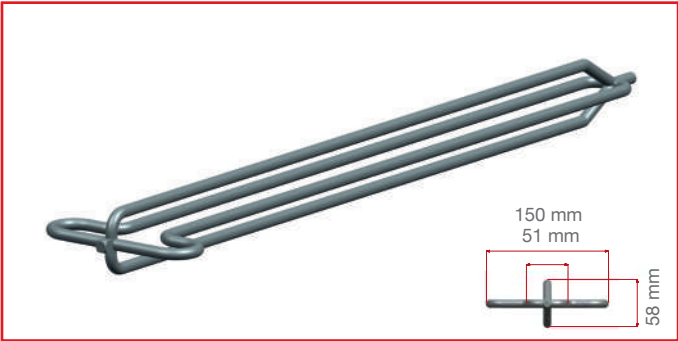
Attrezzo rapido per polli Rocket
