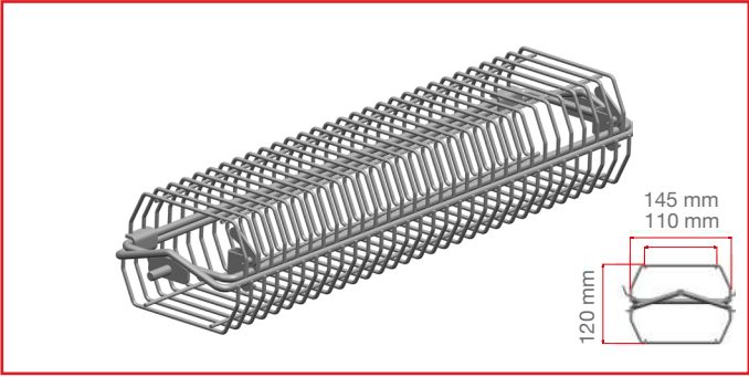
Attrezzo per arrosto Ø 120 mm
