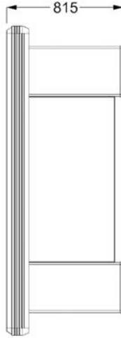
Check Out Counter Without Belt "U" (Lux) Bantsız "U" Yazar Kasa Altı (Lux)
