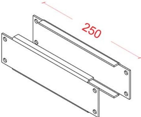
Heavy Duty Rack Back to Back Connection Part Ağır Rack Sırt Sırt Düz Bağlantı Parçası
