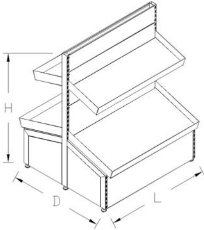
Fruit And Vegetable Middle Unit - ÇR Meyve Sebze Orta Ünitesi - ÇR
