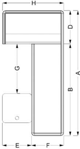
Check Out Counter Without Belt "U" (Lux) Bantsız "U" Yazar Kasa Altı (Lux)
