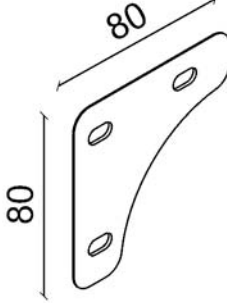
Steel Shelf Corner Triangle Çelik Raf Köşe Üçgen
