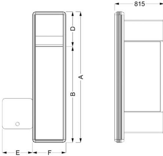
Check Out Counter Without Belt "L" (Lux) Bantsız "L" Yazar Kasa Altı (Lux)
