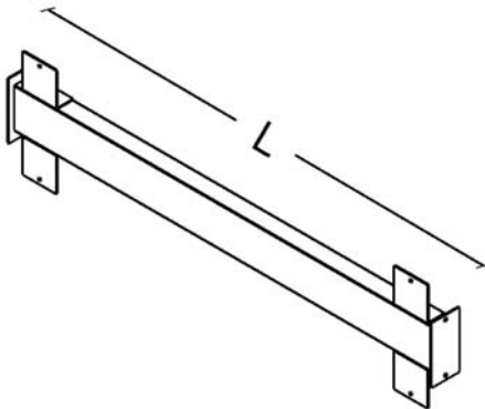
Double Side Depth Connector Çift Taraflı Ara Bağlantı Parçası
