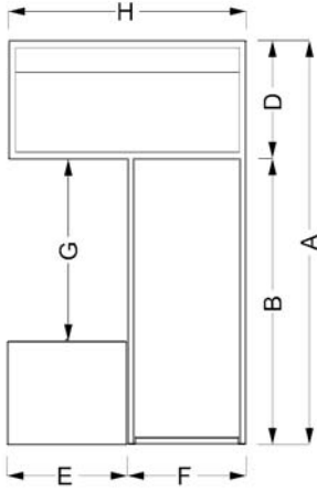
Check Out Counter "U" (Eko) "U" Yazar Kasa Altı (Eko)
