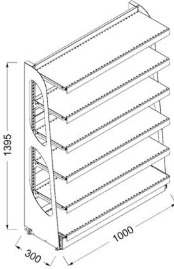
Check Out Stand Kasa Önü Stand
