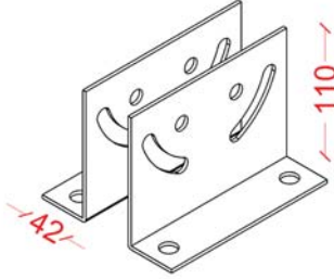
Heavy Duty Rack Elongation Floor Fixer Ağır Rack Gerdirme Yer Bağlantı
