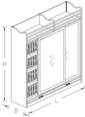
Wooden Bakery Unit Cabinet Ahşap Unlu Mamül Ünitesi (Kapaklı)
