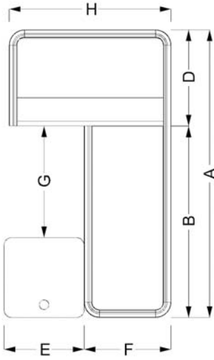
Check Out Counter Without Belt "U" (Eko Lux) Bantsız "U" Yazar Kasa Altı (Eko Lux)
