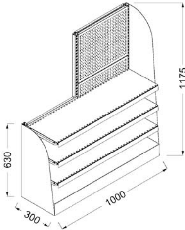
Check Out Stand Kasa Önü Stand
