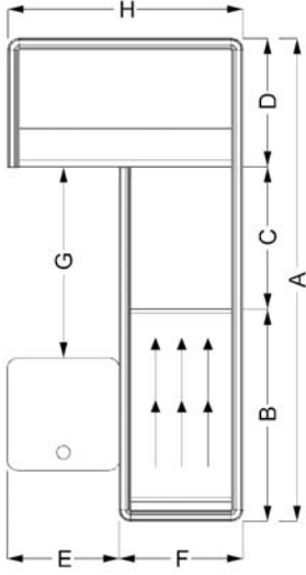
Check Out Counter With Belt "U" (Lux) Bantlı "U" Yazar Kasa Altı (Lux)
